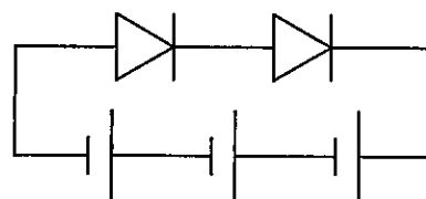
図2 3個の電池と2個のLEDをそれぞれ同じ向きに直列につないだようす
