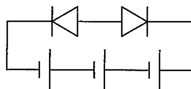
図5 3個の電池と2個のLEDをそれぞれ直列につないだ後、1個のLEDを逆向きにつなぎ変えたようす
