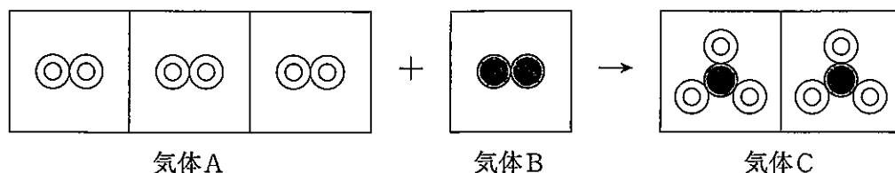
図3 気体Aと気体Bから気体Cができる化学変化
