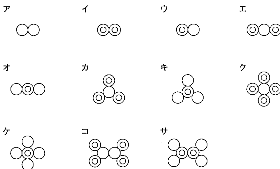
図3 気体Aと気体Bから気体Cができる化学変化
