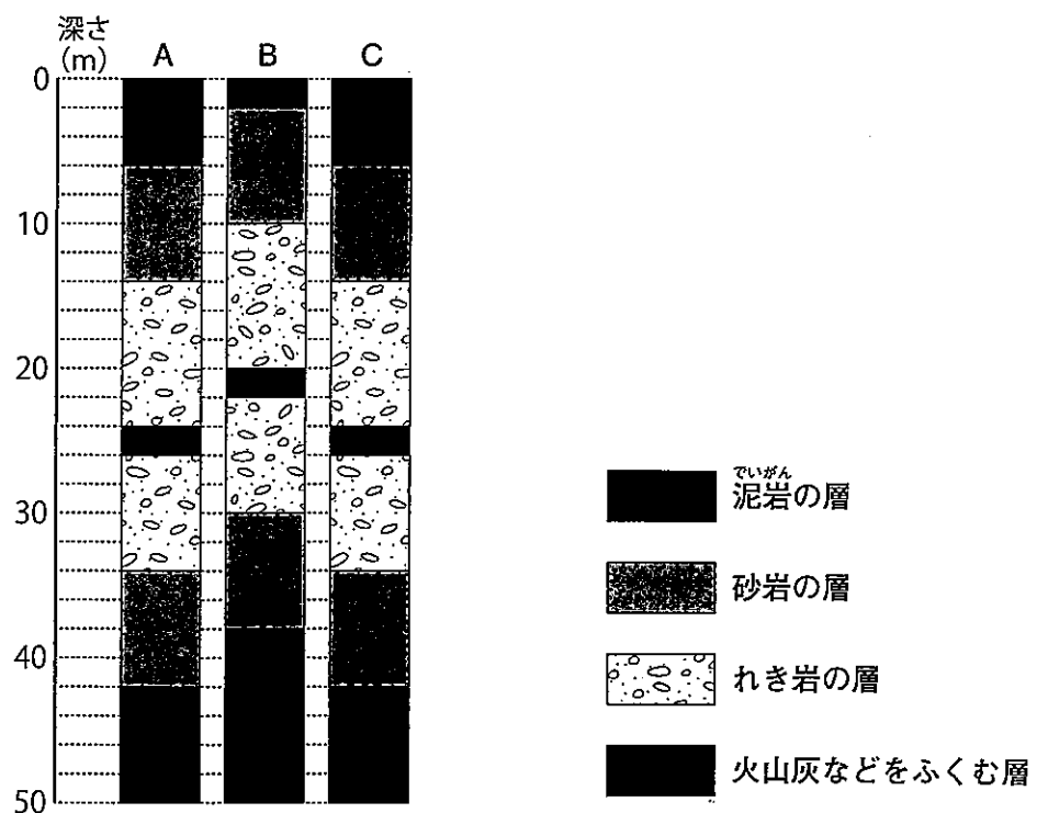
図2 地点A～Cの柱状図
