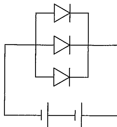
図4 2個の電池を同じ向きに直列につなぎ、3個のLEDを同じ向きに並列につないだようす
