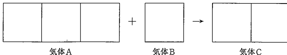
図2 気体A 1.5Lと気体B 0.5Lから気体Cが1Lできる化学変化
