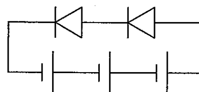
図1 3個の電池と2個のLEDをそれぞれ同じ向きに直列につないだようす
