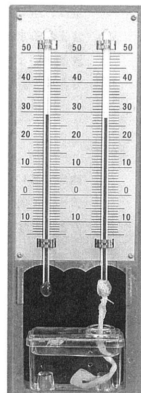
図3 乾湿計
